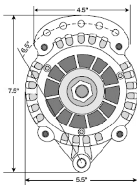
Vorderansicht series 6
